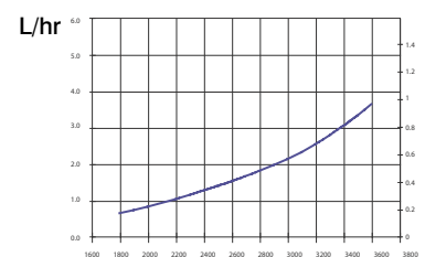
Kraftstoff-Verbrauch in L/hr
